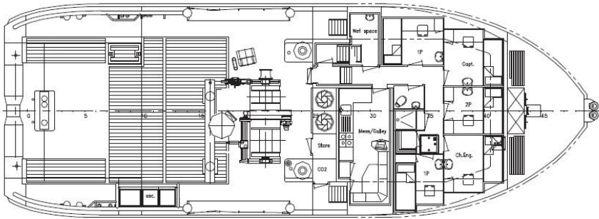
MAINDECK
