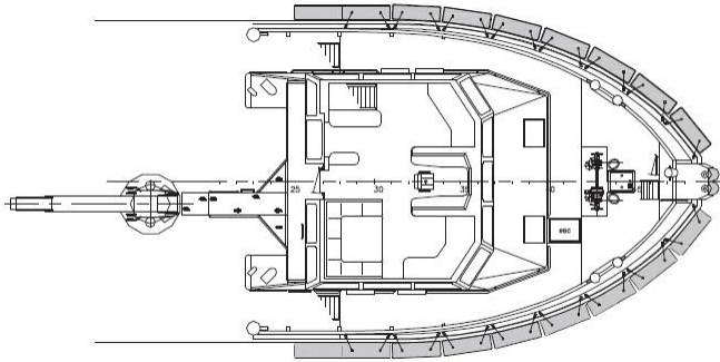
MAINDECK
